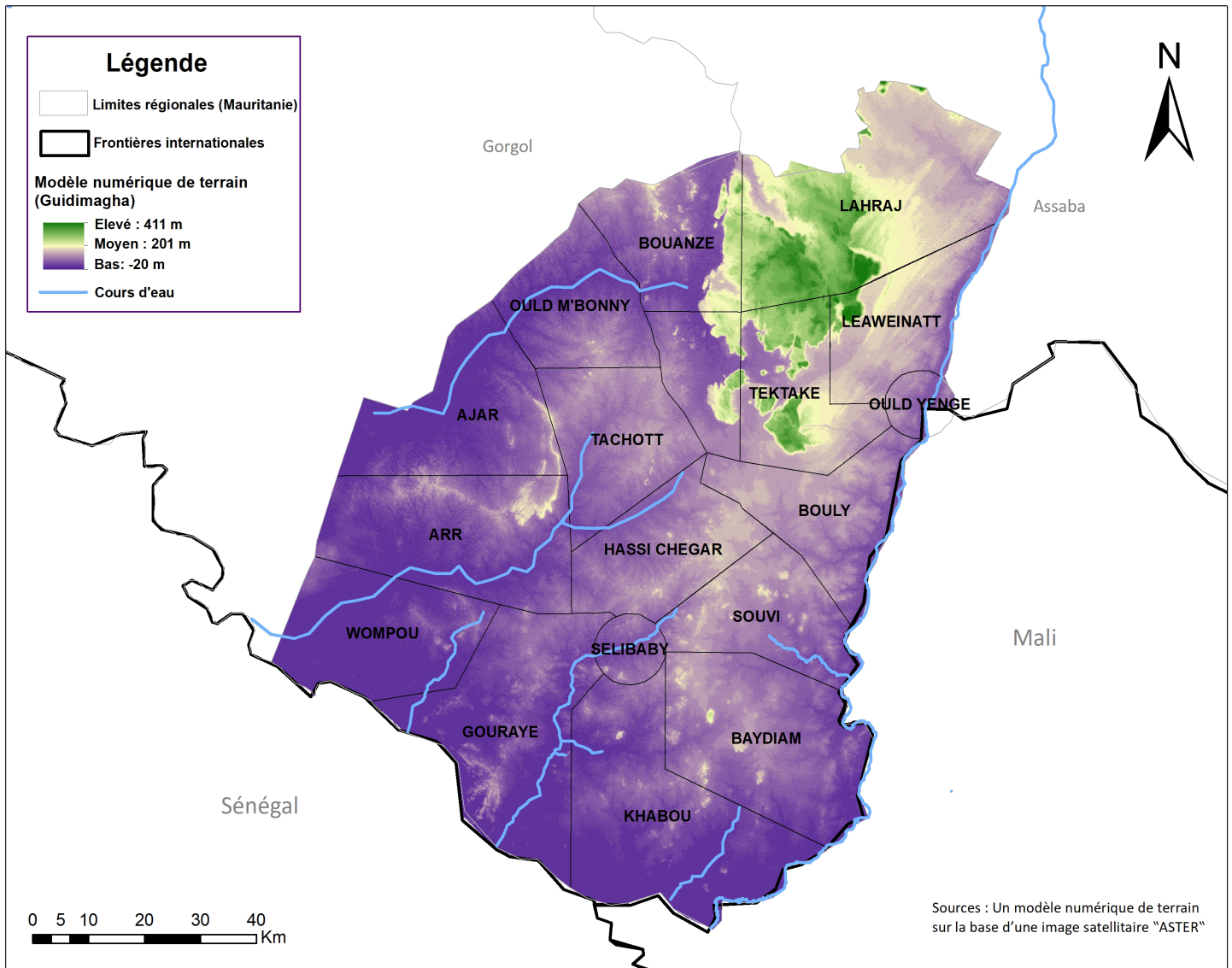
Carte 2: Modèle numérique de terrain de la région de Guidimagha.
