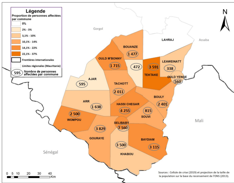
Carte 1: Proportion et nombre de personnes affectées par les inondations, par commune.
