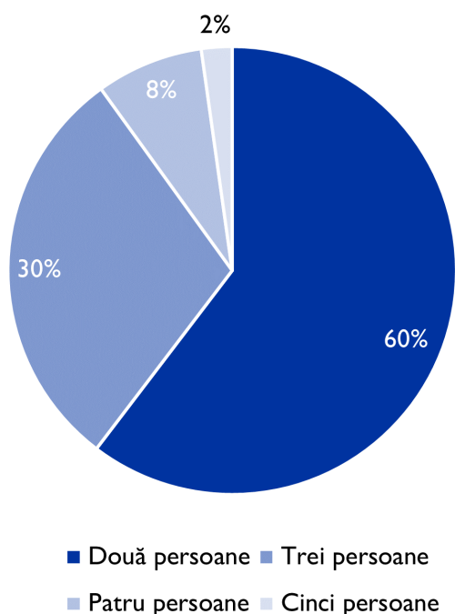
Figura 26: Dimensiunea grupului, (%)
